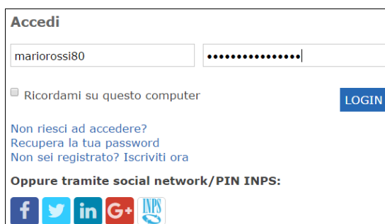
Figura 2 - Login
